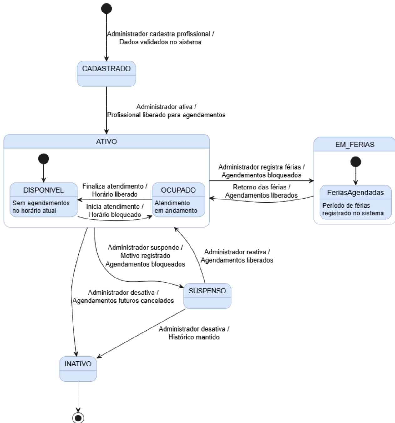
Diagrama de Estados — Profissional
