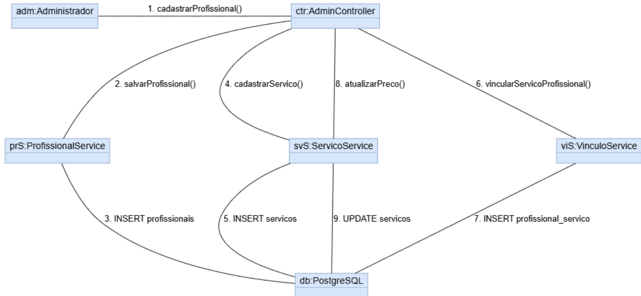
Diagrama de Comunicação — UC-02: Gerenciar Profissionais e Serviços
