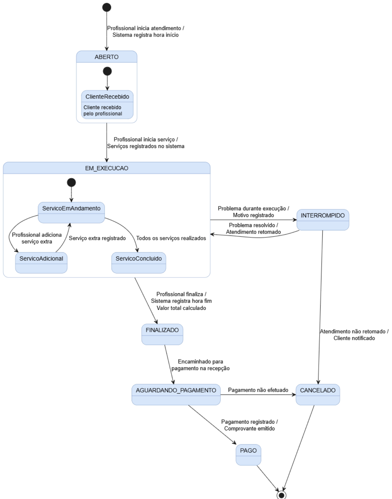
Diagrama de Estados — Atendimento
