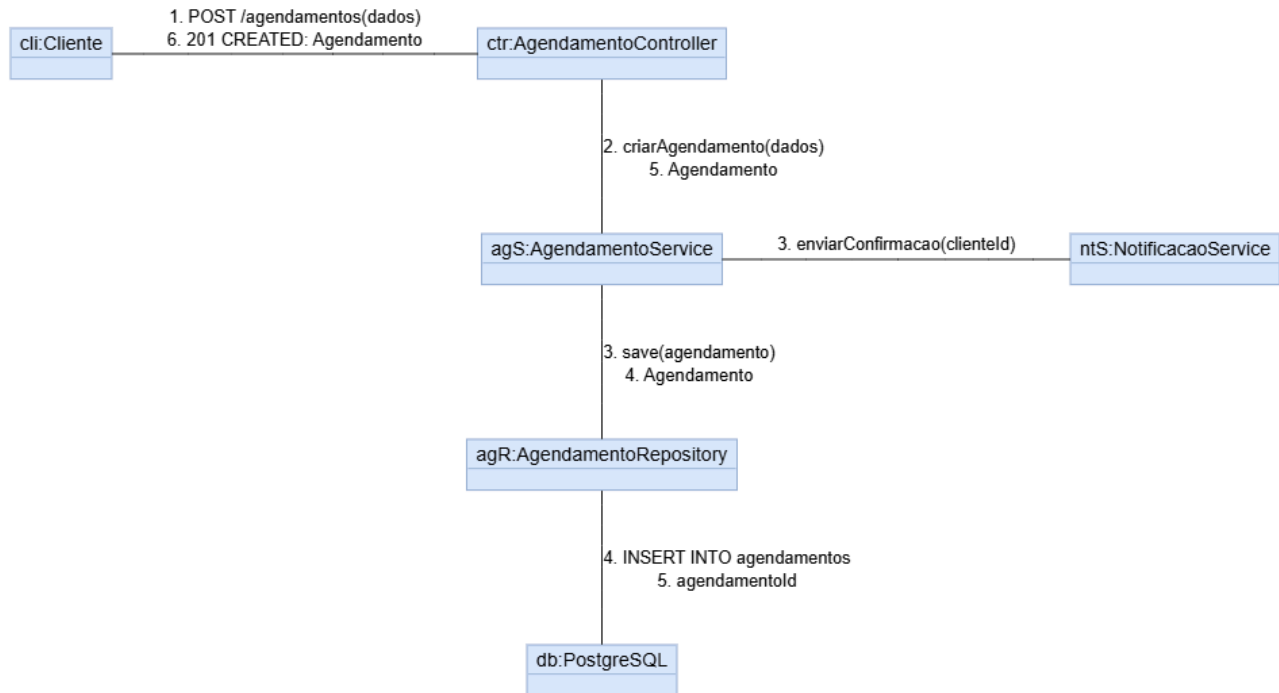
Diagrama de Comunicação — UC-01: Agendar Serviço
