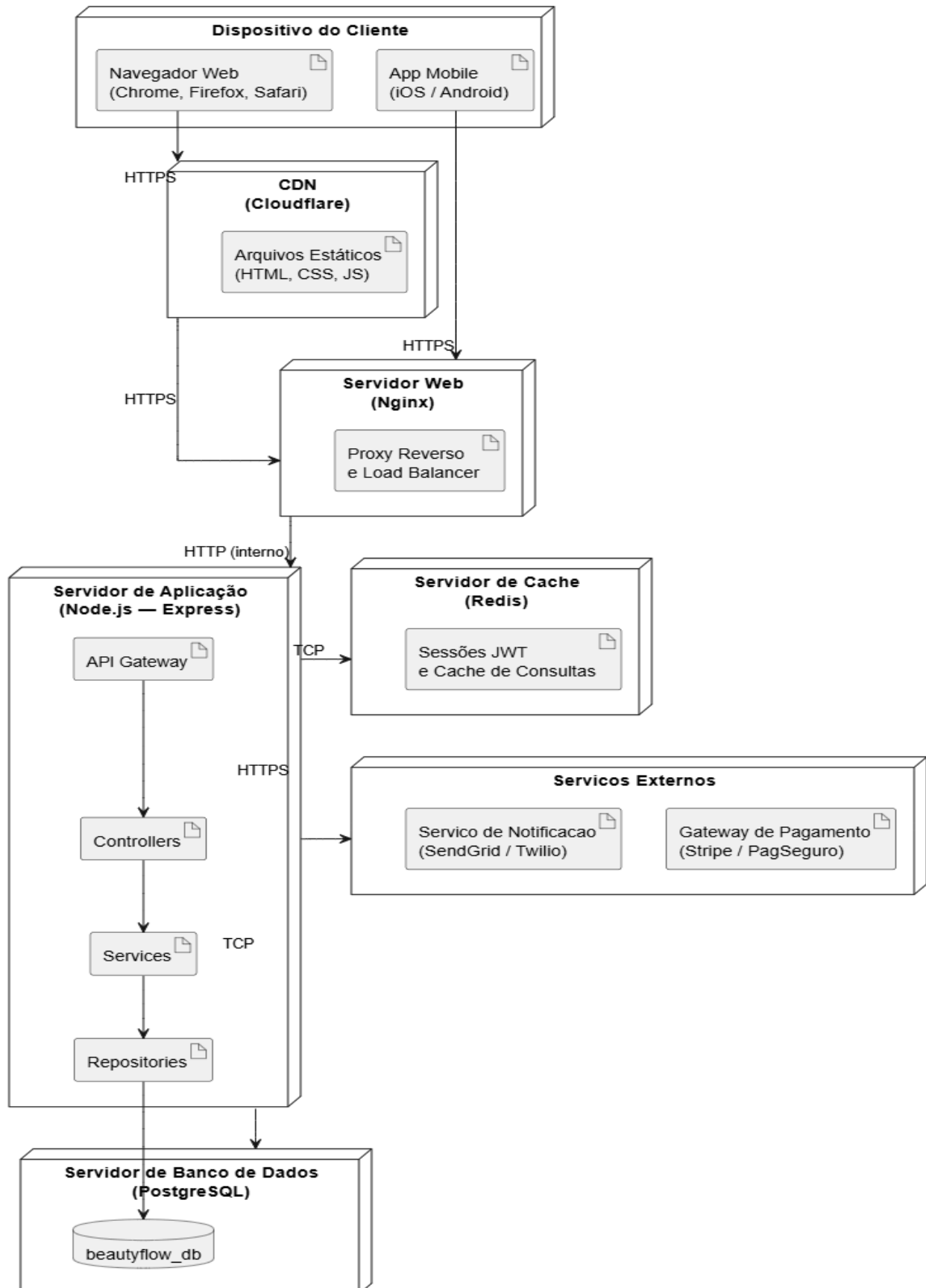
BeautyFlow — Diagrama de Implantação
