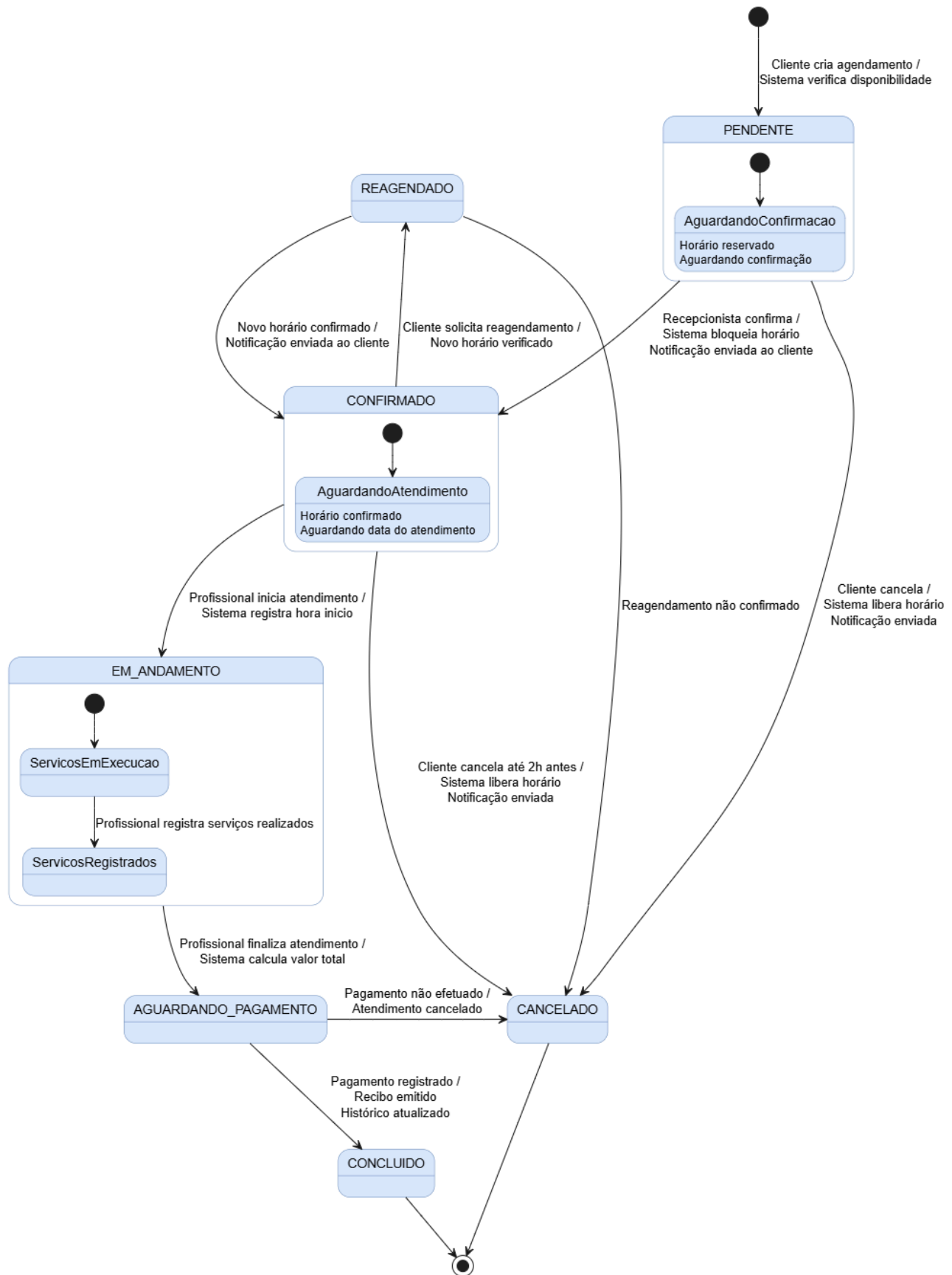
Diagrama de Estados — Agendamento
