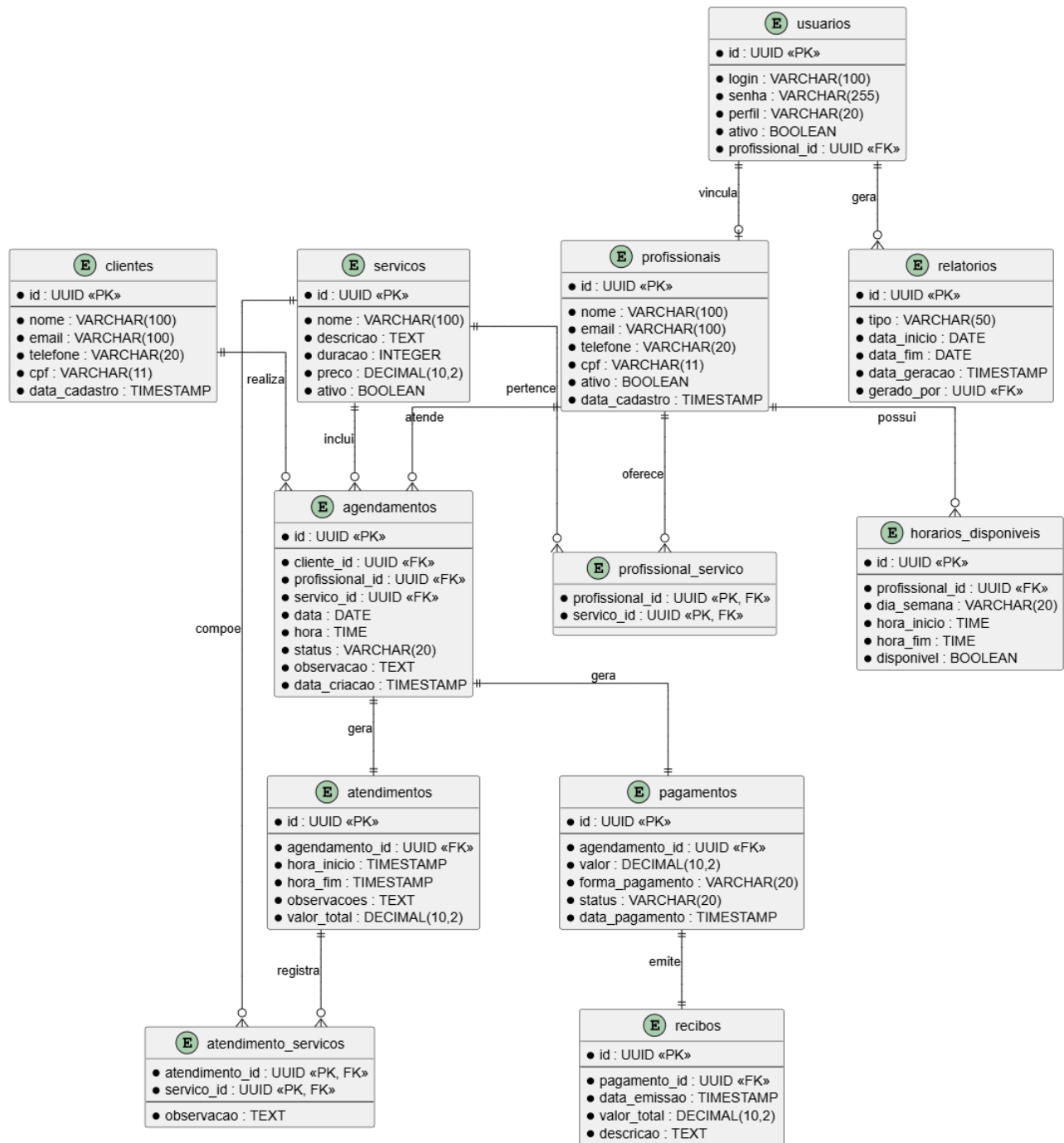
Modelo de Dados — BeautyFlow
