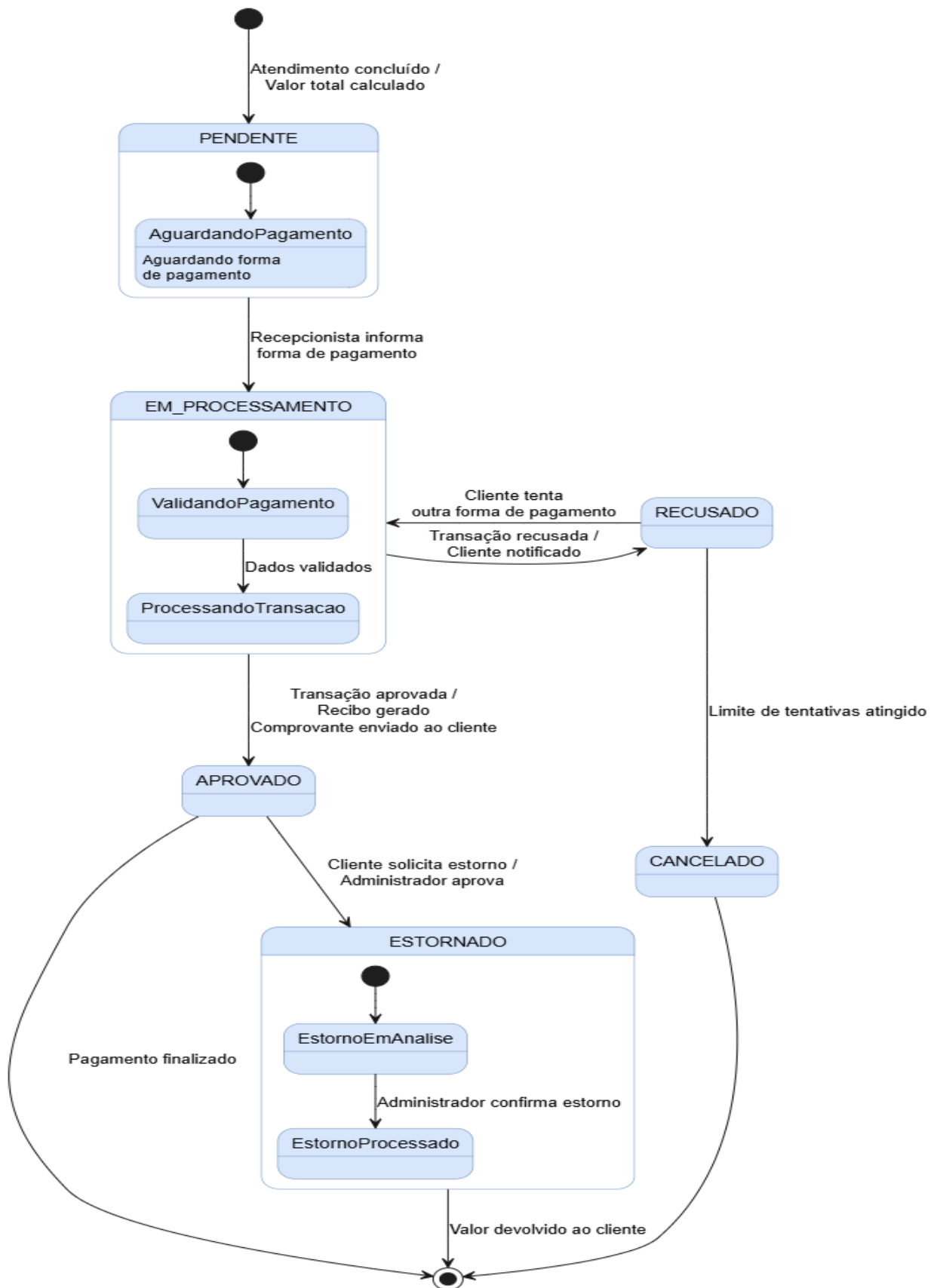
Diagrama de Estados — Pagamento
